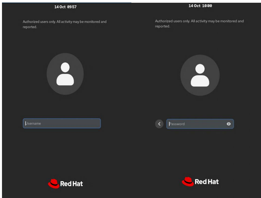
Kuva 3. VISU-linux kirjautumisikkuna.
